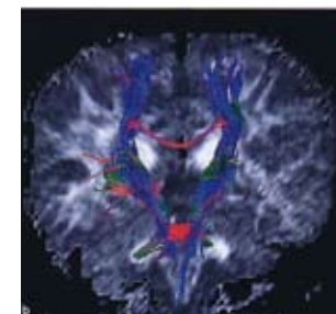
Fig.3-27 – Traçage des fibres à partir de l'algorithme de reconstruction du tenseur. Représentation du corps calleux (a) et du faisceau pyramidal (b).
